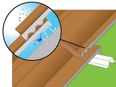
สันรางด้านข้าง ป้องกันการรั่วซึมระหว่างแผ่น
