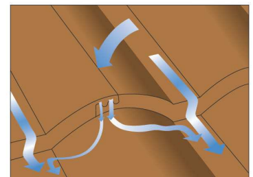
บัวดักน้ำ 3 ชั้น 2 ร่องลึก ป้องกันน้ำฝนไหลย้อนกลับเข้าใต้หลังคา
